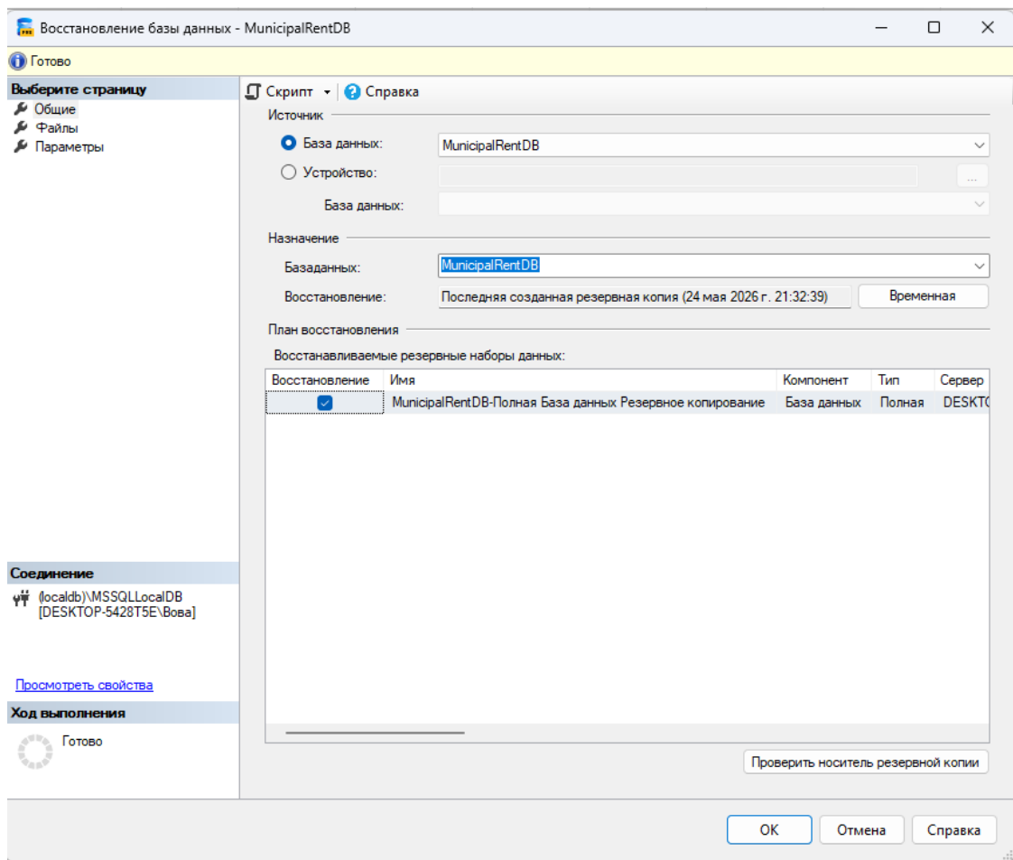
Рисунок 13 - Восстановление БД
