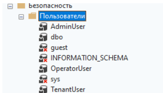
Рисунок 5 - Пользователи БД
