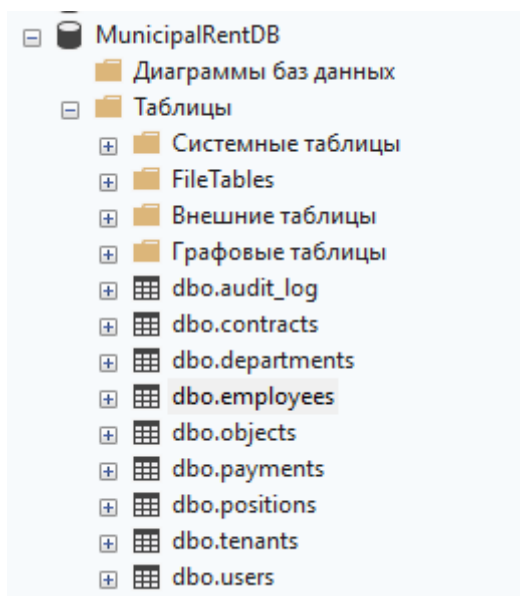
Рисунок 4 - Таблицы БД
