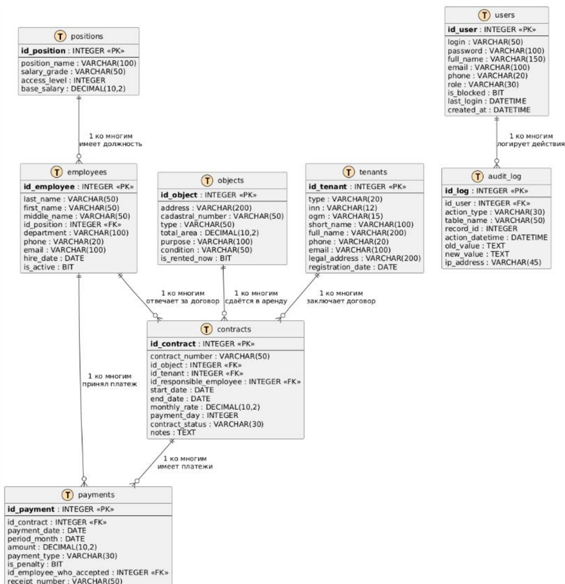
Рисунок 1 - ER-диаграмма
