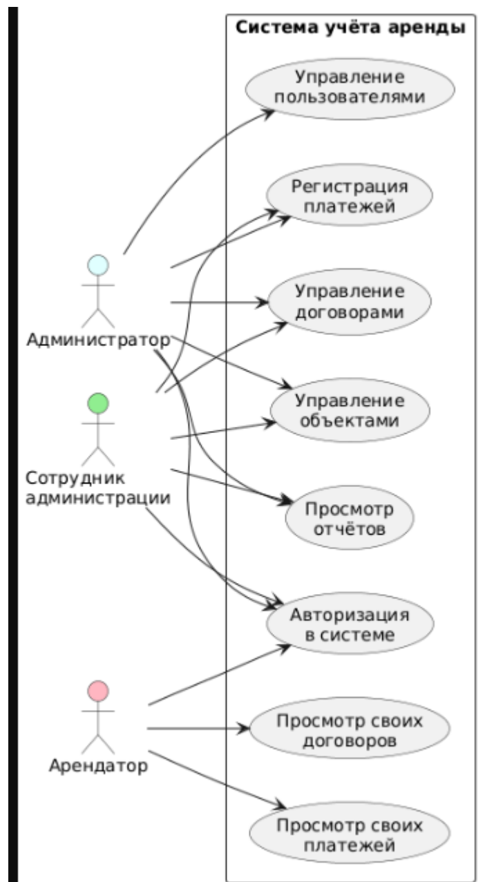
Рисунок 2 - UML-диаграмма
