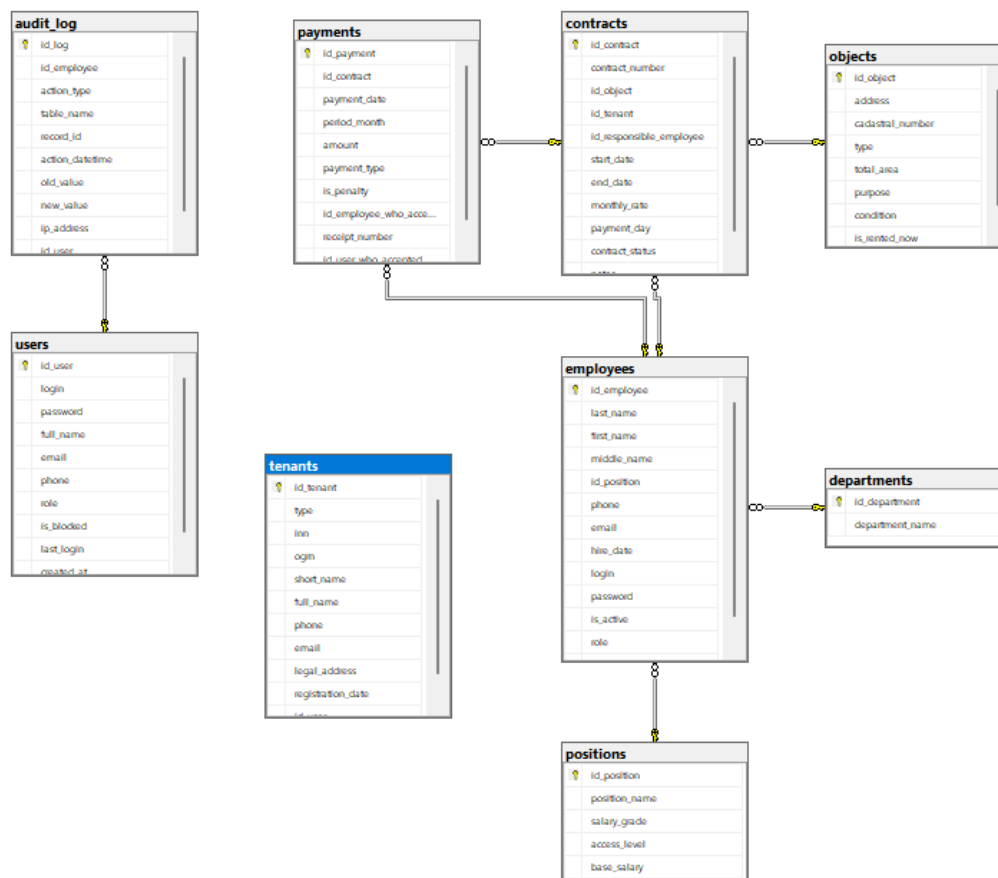
Рисунок 3 - Диаграмма БД
